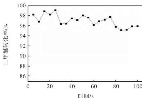
图6 Pt-Ce/HZSM-5 催化燃烧二甲醚的稳定性分析
