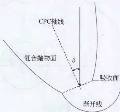
(a) 设计图
