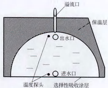
图 4 集热器水箱示意图
