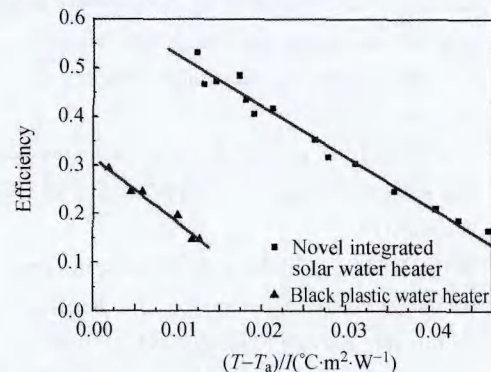
图 7 新型和传统黑色塑料袋闷晒式太阳能热水器的瞬时效率曲线
